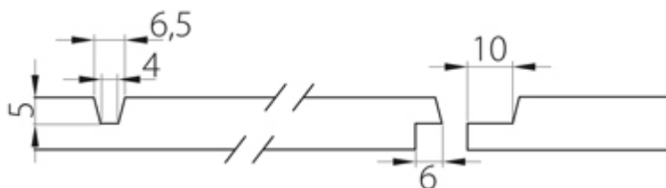
Profil U
