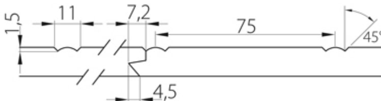
Profil W
