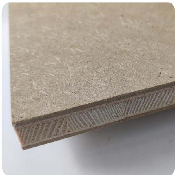
Construction 5 plis pour le format 2800 x 1850
